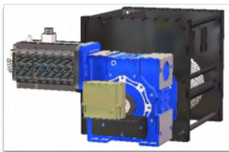
一体式单吊点自动排绳升降机
